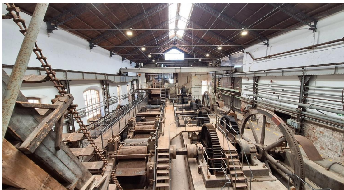
Azucarera El Pilar, nave del tren de molinos, Motril (Granada)
